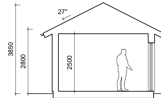
SEKTION A-A 1:100
