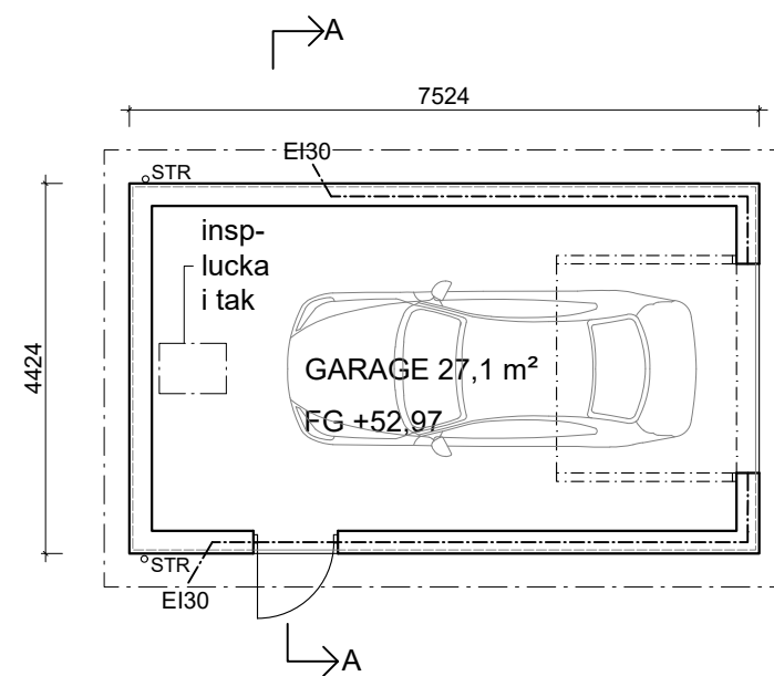
PLAN 1:100
