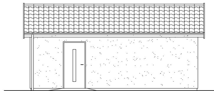
FASAD MOT SÖDER 1:100
