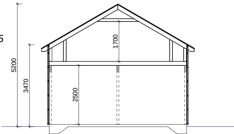
SEKTION A/A
