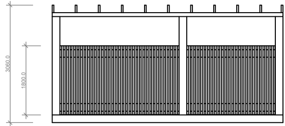
FASAD MOT SÖDER, 1:100
