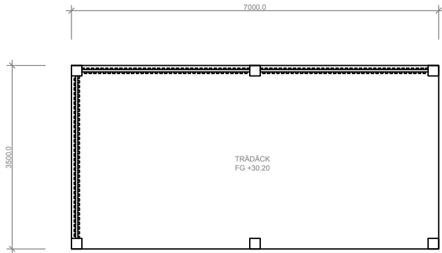
PLAN 1, 1:100
