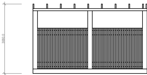
FASAD MOT SÖDER, 1:100
