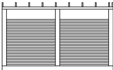
FASAD MOT NORR, 1:100
