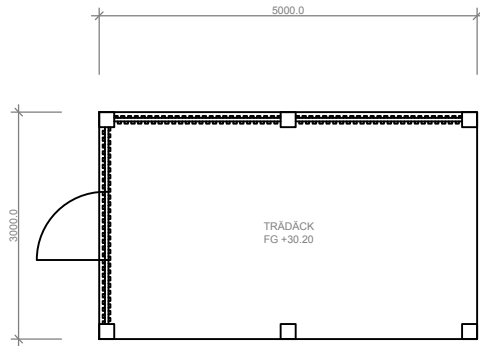
PLAN 1, 1:100
