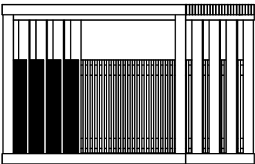
FASAD MOT NORR, 1:100
