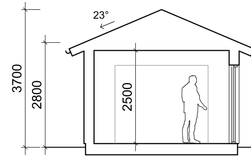
SEKTION A-A 1:100
