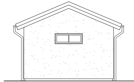
FASAD MOT SÖDER 1:100
