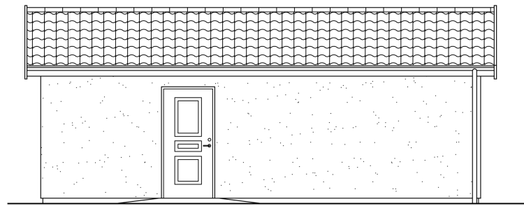
FASAD MOT ÖSTER 1:100
