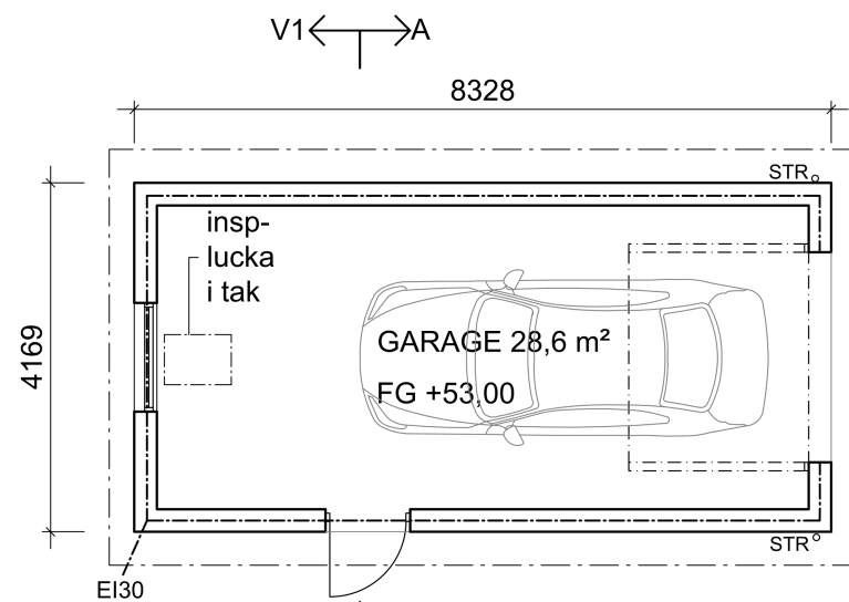
PLAN 1:100
