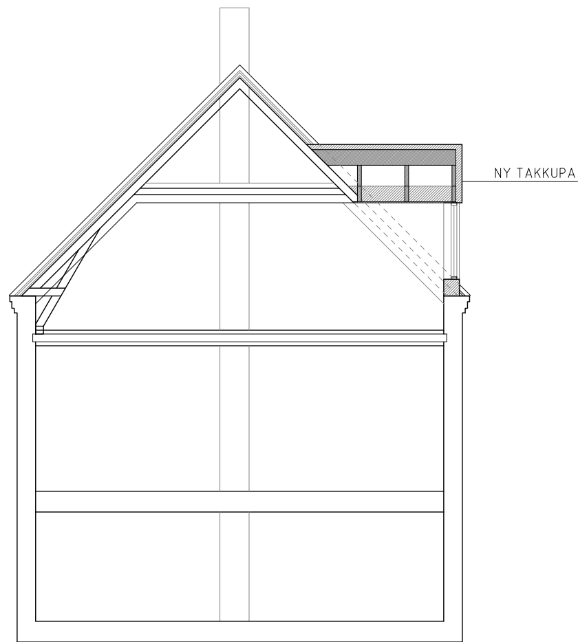
SEKTION a-a
