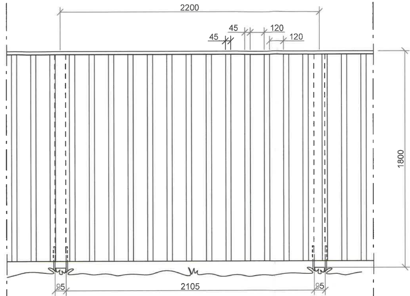
elevation plank h.1800 mm
