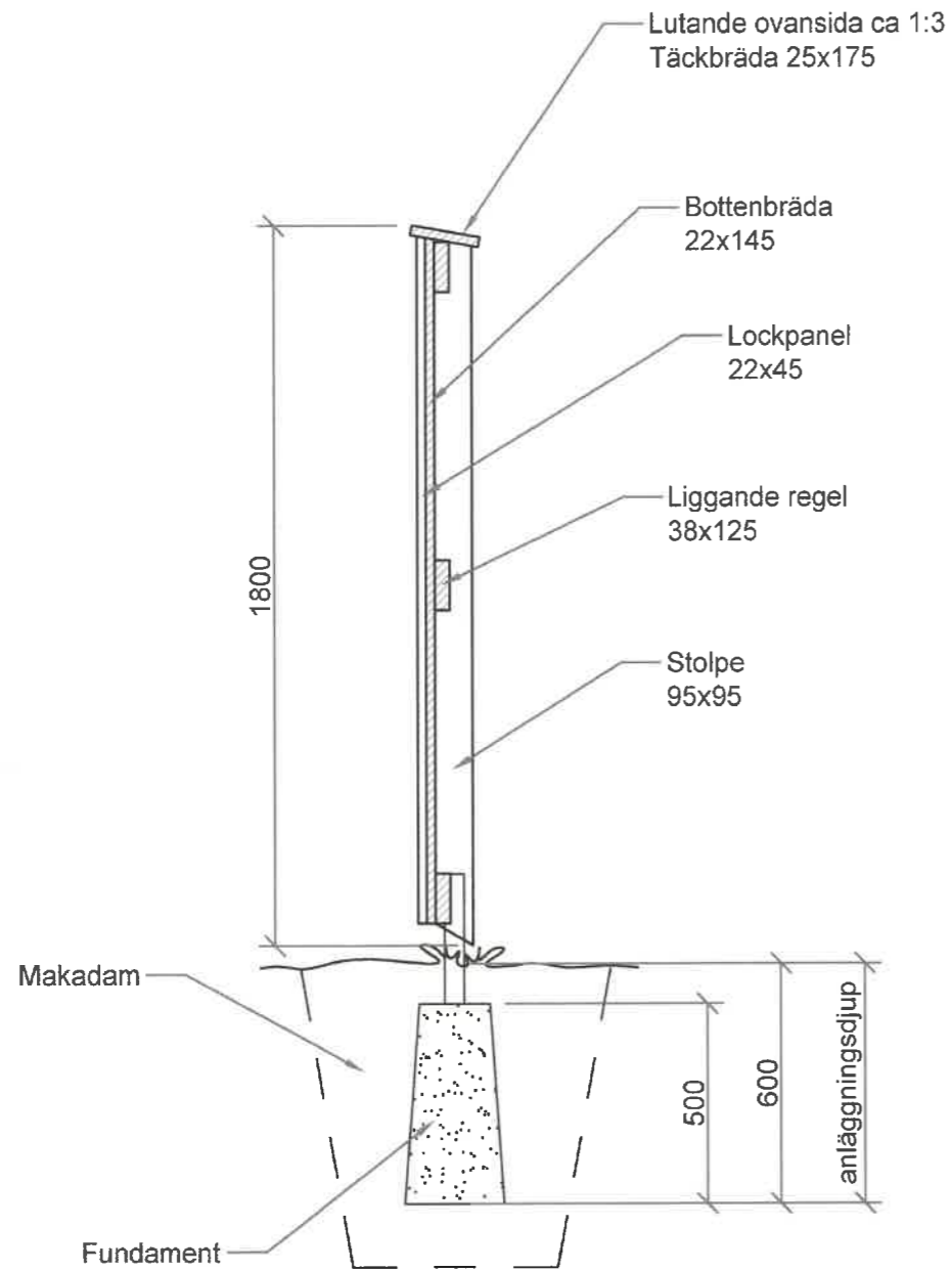
sektion plank h.1800 mm
