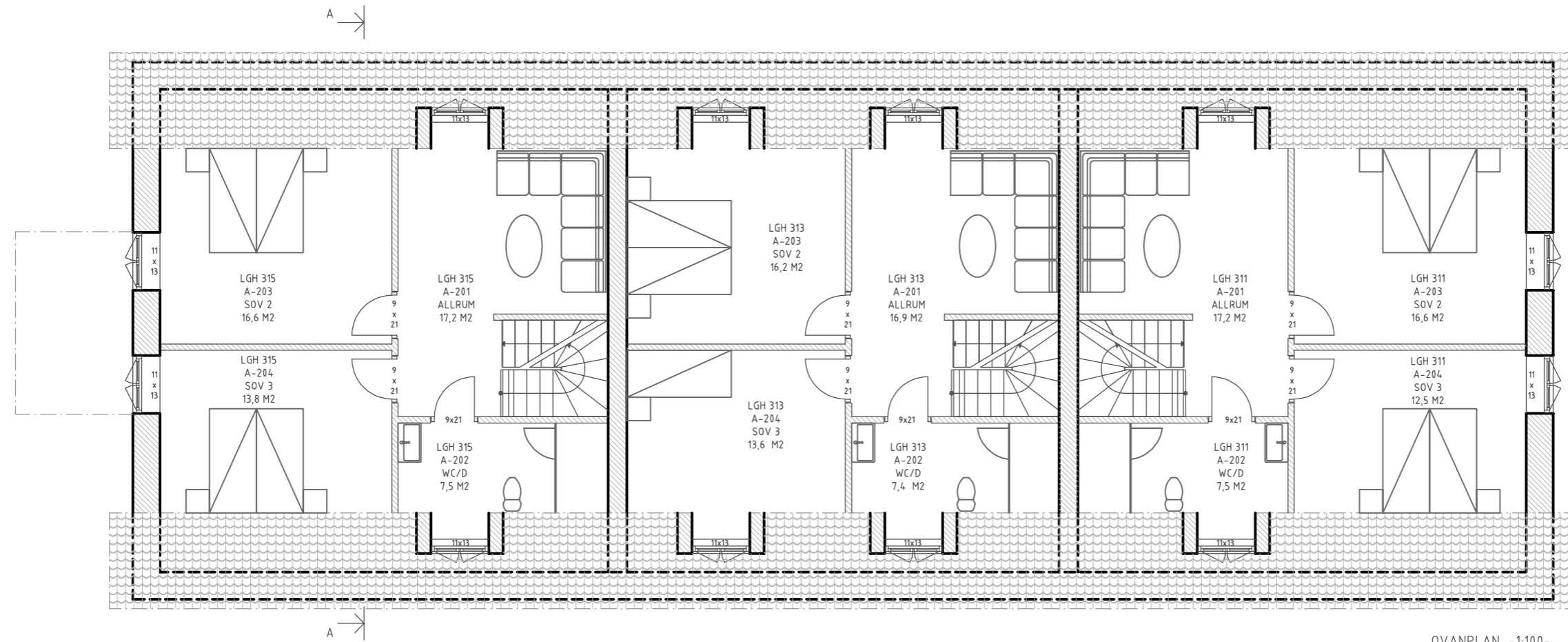
OVANPLAN -1:100-
